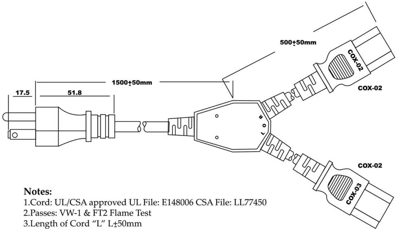
Plug:COX-01
